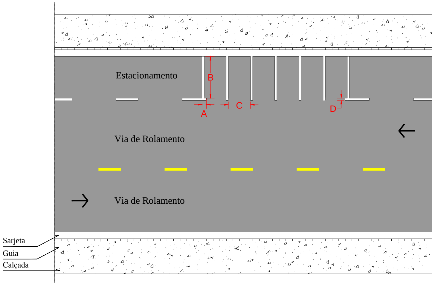
Marcação de área de estacionamento para motocicletas
